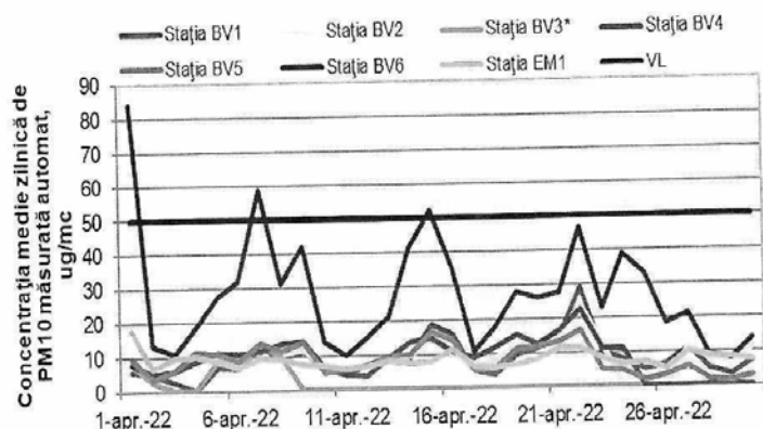
Figura 1.1.2.4.1. Evoluția mediilor zilnice de PM 10 în luna aprilie
