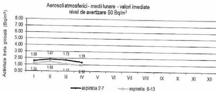
Fig. 1.2.1. Activitatea beta globală pentru aerosoli atmosferici
