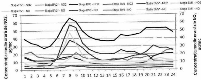
Figura 1.1.2.2.2. Ciclul zilnic al NO 2 și NO
