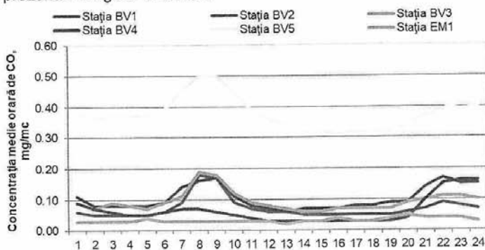
Figura 1.1.2.5.2. Ciclul zilnic al CO
