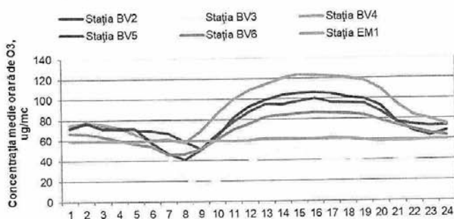
Figura 1.1.2.3.2. Ciclul zilnic al ozonului
