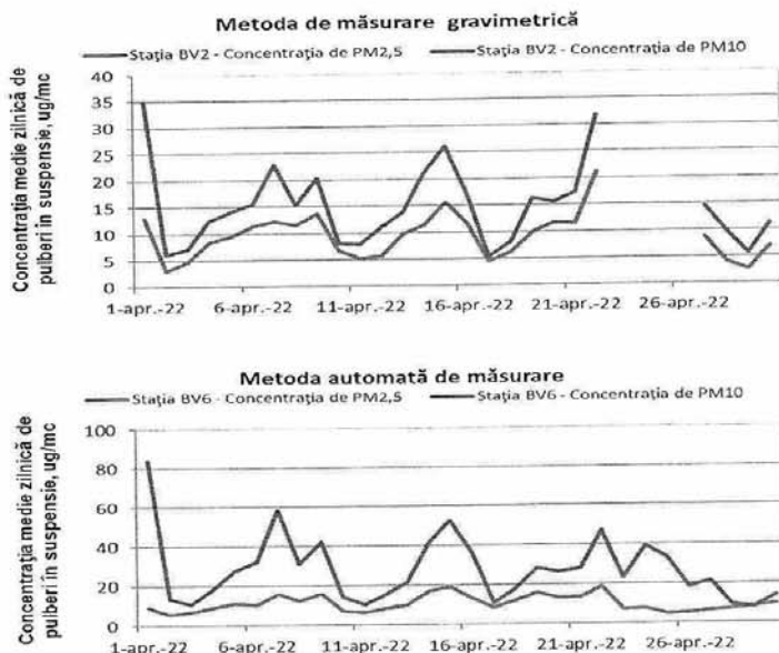
Figura 1.1.2.4.4 Evoluția mediilor zilnice de PM 2,5 și PM10 în luna aprilie
