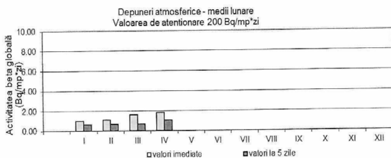
Fig. 1.2.4. Activitatea beta globală pentru depuneri atmosferice
