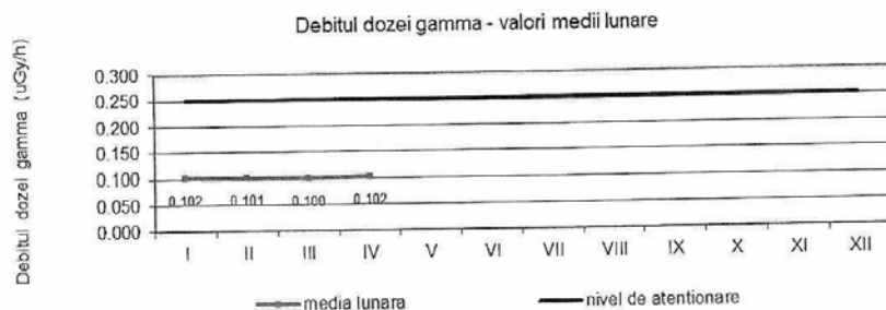
Fig. 1.2.3. Debitul dozei gamma în aer
