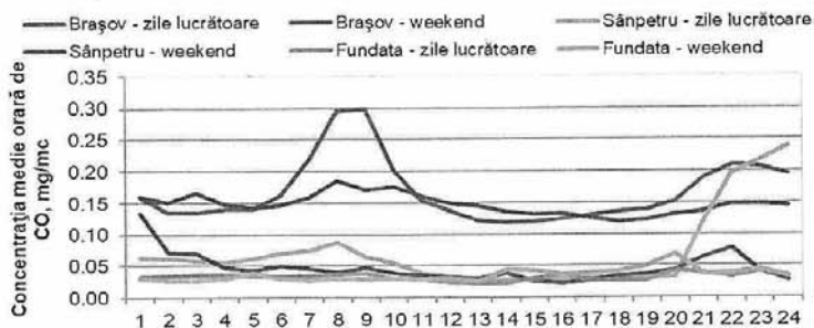
Figura 1.1.2.5.3. Ciclul zilnic al CO în timpul săptămânii
