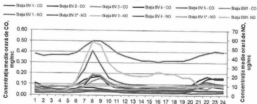
Figura 1.1.2.2.4. Ciclu zilnic al NO și CO
